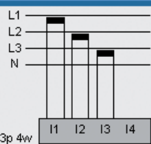
Abb. Beispiel für die Strommessung über 3 Stromwandler in einem 3 Phasen 4 Leiter Netz.
