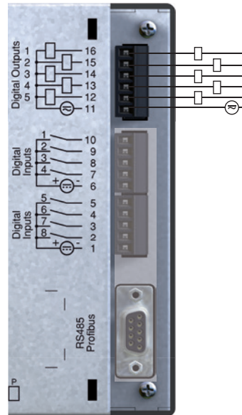
Abb. Anschluss digitale Ausgänge.
