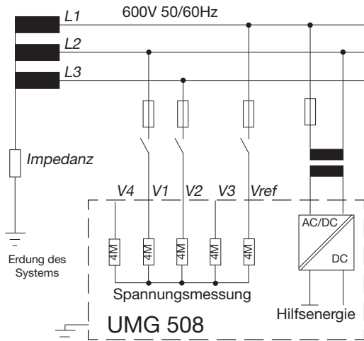
Abb. Prinzipschaltbild, UMG 508 im IT-Netz ohne N .
