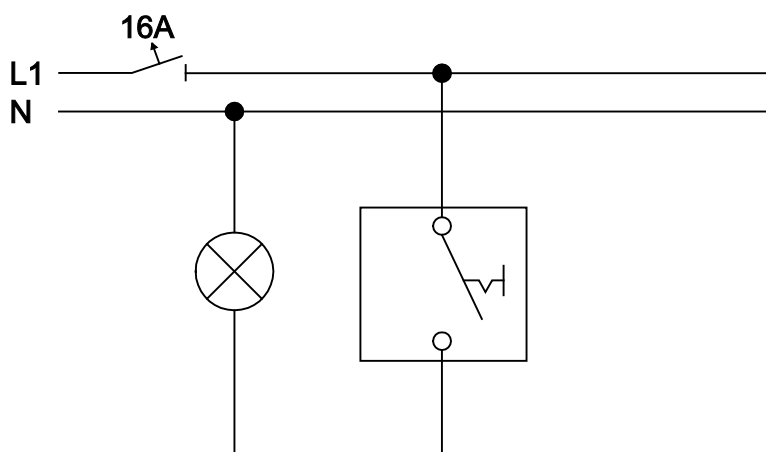
Afb. 2: Uitschakeling
