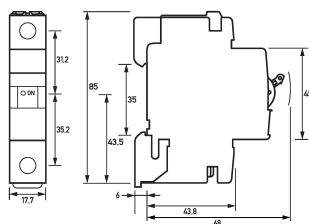
Maßzeichnung Gruppenansicht
