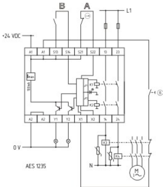
Schaltungsbeispiel
