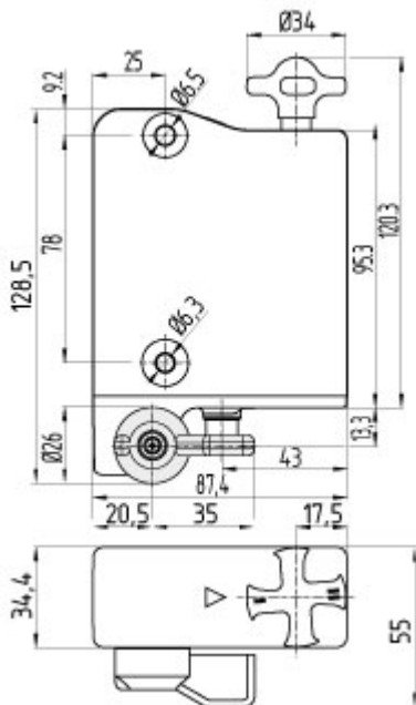
Maßzeichnung (Grundgerät)
