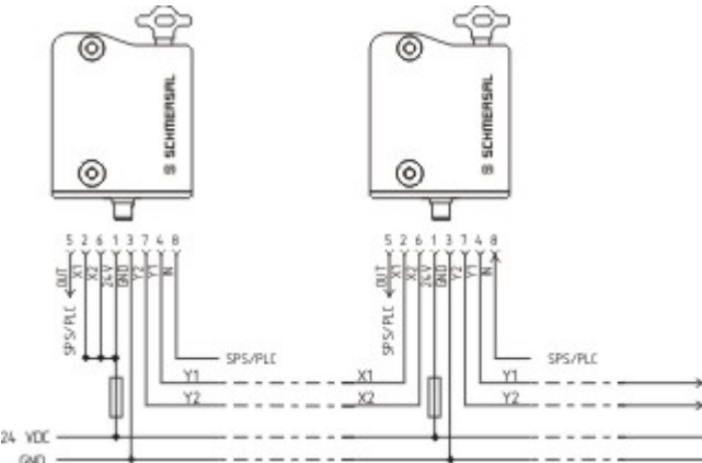
Schaltungsbeispiel
