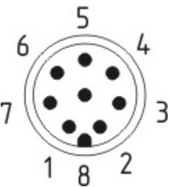
Polbild
