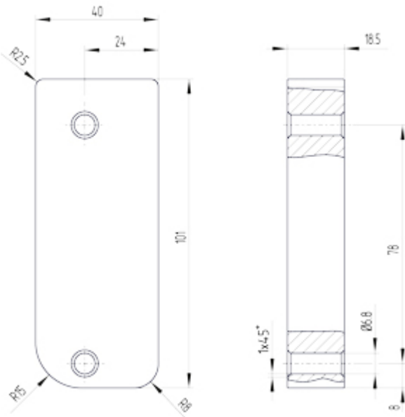
Maßzeichnung (Grundgerät)
