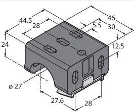
LMBWLS27U 3094775 Universal-Montagehalterung für WLS27
