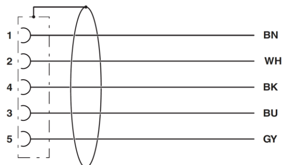
Leitung
