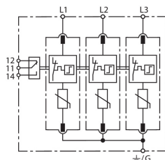
Prinzipschaltbild DG MU 3PY 600 3W+G R
