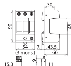
Maßbild DG MU 3PY 600 3W+G R
