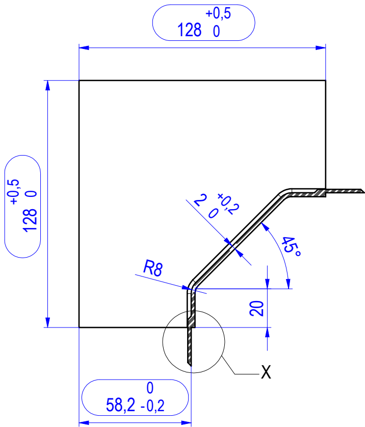
SCHNITT A-A
