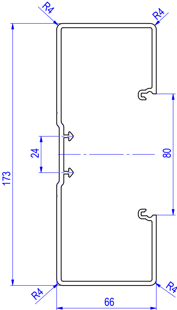
Lichter Querschnitt / cross section : 9750 mm²
