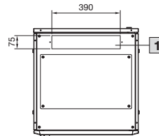
Draufsicht, Breite 800 mm/Tiefe 800 mm
