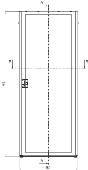
Vorderansicht
