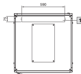
Draufsicht, Breite 800 mm/Tiefe 800 mm
