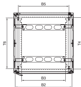
Schnitt B – B
