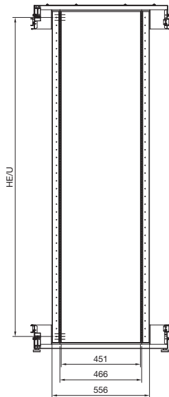
Schnitt B – B
