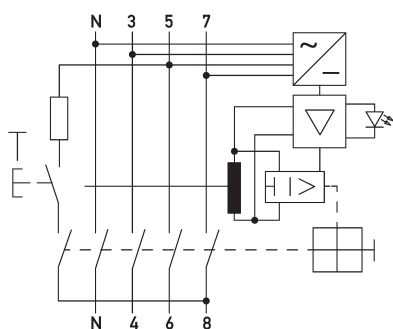
Schaltungsbeispiel Fehlerstromschutzschalter DFS 4 063-4/0,10-PV
