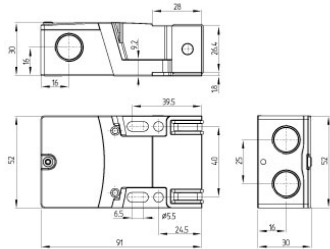
Maßzeichnung (Grundgerät)
