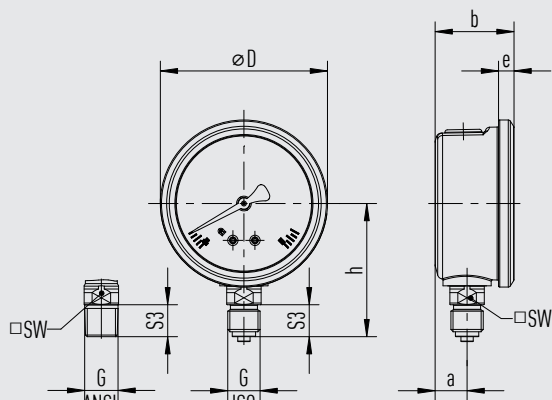
NG 50 [2"] und NG 63 [2 ½"], Anschluss radial unten
