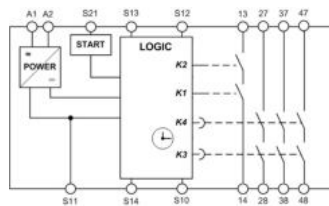
Abb. 1 Blockschaltbilder: SR4C (1unverz./3verz.);
