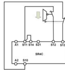
Abb. 7: Zweikanalige Schliebeschützgitter-Überwachung mit Querschuss- und Erdschluss-Überwachung. (Kategorie 4, bis PL e / SIL 3)
