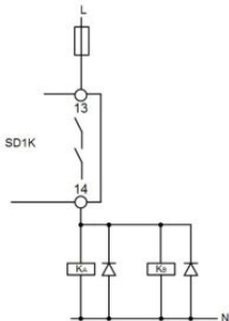
Abb. 8 Sicherer Relaiskontakt
