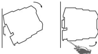
Abb. 3 Montage / Demontage
