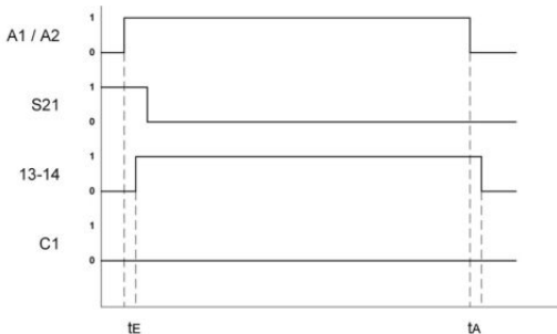
Abb. 10 Zeitdiagramm - SD1K mit Rückführkreis an S21
