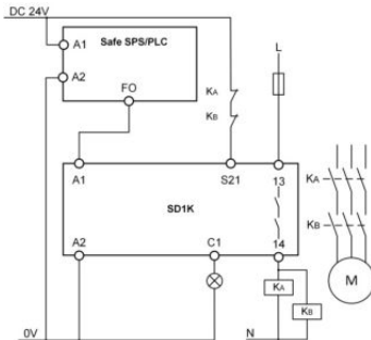
Abb. 2 Kontaktverstärkung und Testpulsfilterung
