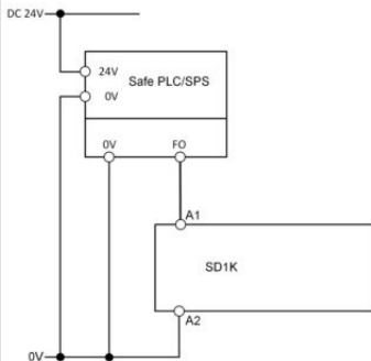
Abb. 7 Ansteuerung SD1K über Safe PLC/SPS
