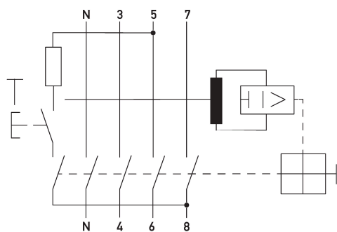
Schaltungsbeispiel Fehlerstromschutzschalter DFS 4 025-4/0,03-F
