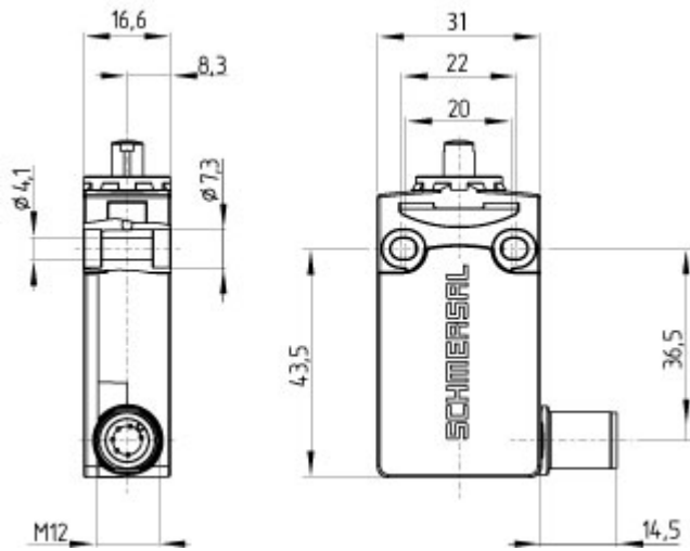
Maßzeichnung (Grundgerät)
