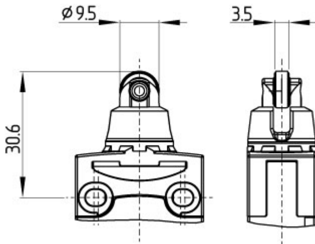
Maßzeichnung (Betätiger)
