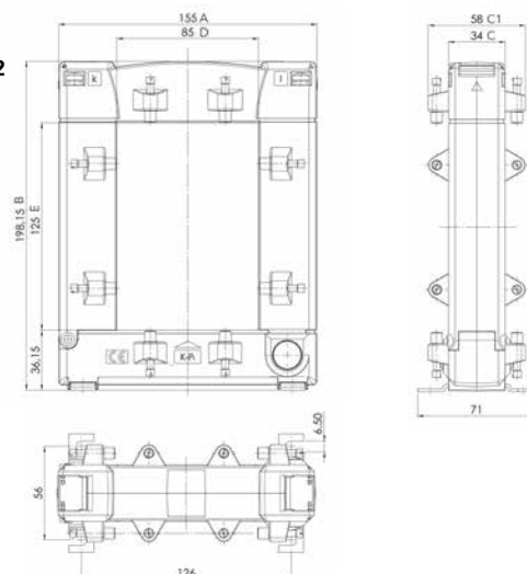
KBU 812
