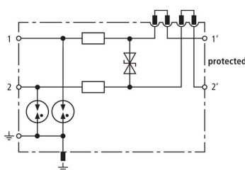
Prinzipialschaltbild DCO SD2 MD 24
