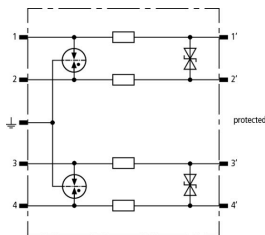
Prinzipschaltbild BSP M4 BD 24
