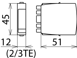
Maßbild BSP M4 BD 24
