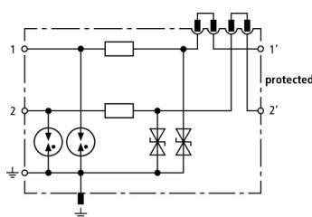
Prinzipschaltbild DCO SD2 ME 48
