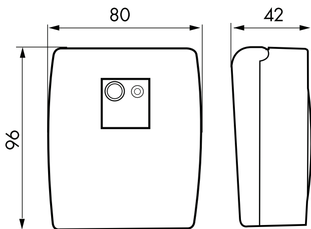
Bemaßung 92369
