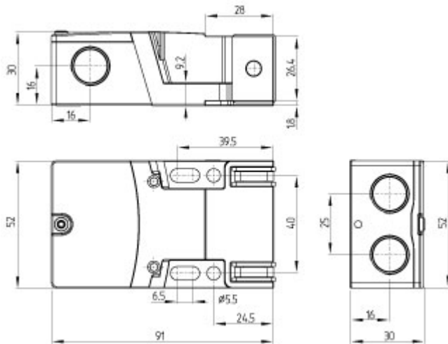
Maßzeichnung (Grundgerät)
