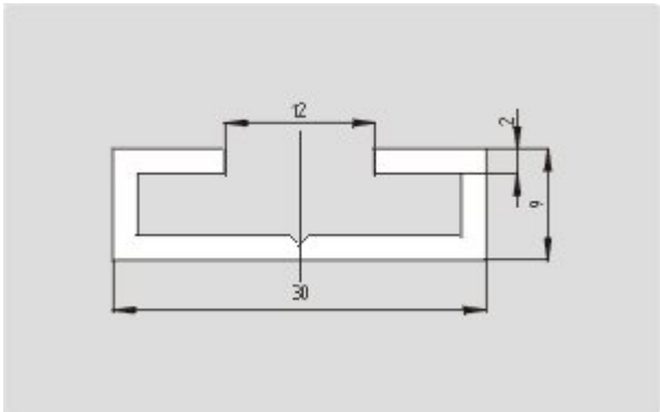
Maßzeichnung (Grundgerät)
