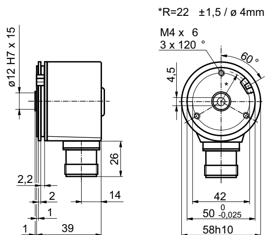
BHF Gerätestecker radial
