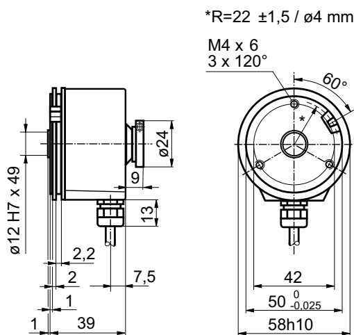
BHG Kabel radial
