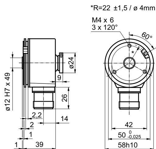
BHG Gerätestecker radial
