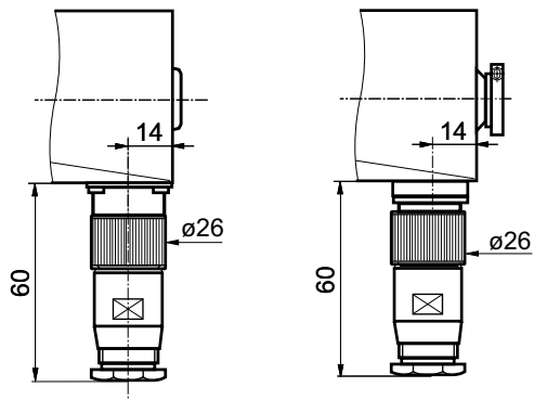
BHF/BHG Steckerabmessungen
