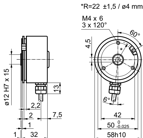
BHF Kabel radial
