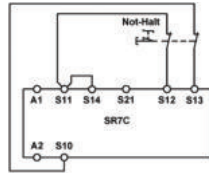
Abb. 4: Zweikanalige Not-Halt-Schaltung mit Querschuss- und Masseschluss-Überwachung (Kategorie 4, bis PL e / SIL 3)
