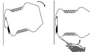
Abb. 2 Montage / Demontage
