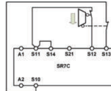
Abb. 6: Einkanalige Not-Halt-Schaltung mit Masseschluss-Überwachung. (Kategorie 1, bis PL c / SIL 1)
