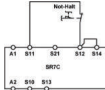
Abb. 6: Einkanalige Not-Halt-Schaltung mit Masseschluss-Überwachung. (Kategorie 1, bis PL c / SIL 1)
