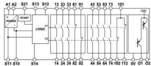
Abb. 1 Blockschaltbild SR7C
