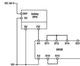
Abb. 10: Anschluss an fehlersichere Steuerung (Kat. 4, bis PL e / SIL 3)
