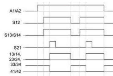
Abb. 2 Zustandsdiagramm SR3E mit man. Start
