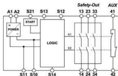
Abb. 1 Blockschaltbild SR3E
