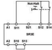
Abb. 5: Zweikanalige Not-Halt-Schaltung mit Querschuss- und Massechluss-Überwachung (Kat. 4, bis PL e / SIL 3)
