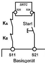
Abb. 7: Rückführkreis mit man. Start
