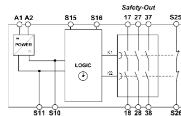
Abb. 1 Blockschalbild SRTC
