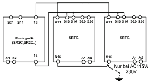
Abb. 7: Rückführkreis mit man. Start
