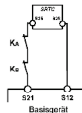
Abb. 8: Rückführkreis mit Auto-Start
