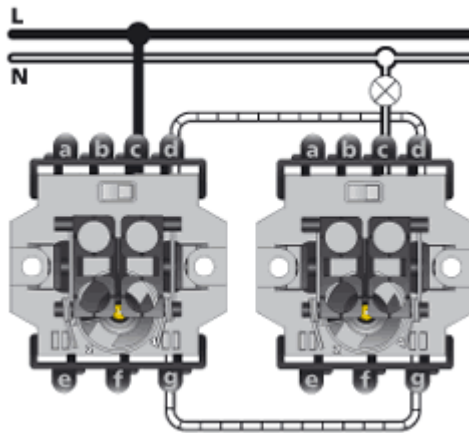
Wechselschaltung
