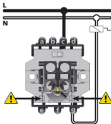
Taster Öffner
