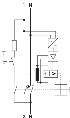
Schaltungsbeispiel FI-/LS-Kombinationen DRCBO 4 B13/0,03/1N-B+
