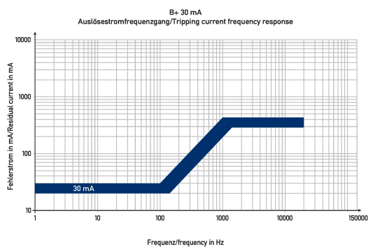
Diagramme FI-/LS-Kombinationen DRCBO 4 B13/0,03/1N-B+
