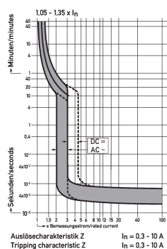
Diagramme Leitungsschutzschalter DLS 6i Z10-2
