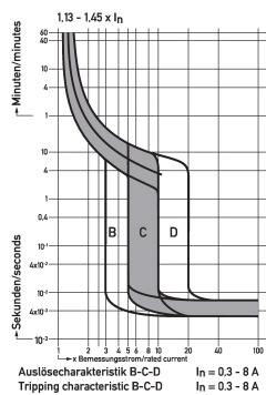
Diagramme Leitungsschutzschalter DLS 6hsl B6-1
