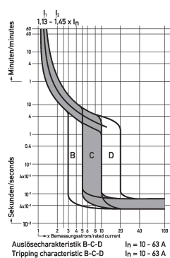
Diagramme Leitungsschutzschalter DLS 6hsl C20-1
