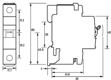
Maßzeichnung Leitungsschutzschalter DLS 6hsl C20-1
