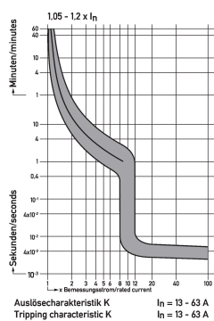
Diagramme Leitungsschutzschalter DLS 6i K16-3
