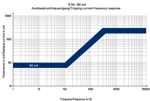
Diagramme Fehlerstromschutzschalter DFS 4 080-4/0,10-B SK
