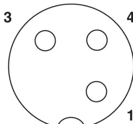
Polbild Buchse M12, 3-polig, A-kodiert, Ansicht Buchsenseite
