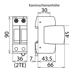
Maßbild DG S PV SCI 150
