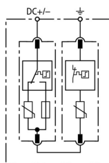
Prinzipschaltbild DG S PV SCI 150
