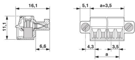
Maßzeichnung
