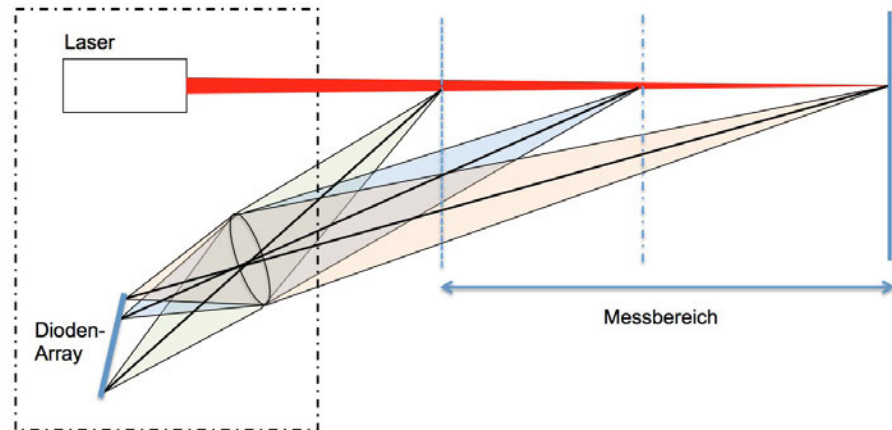
Funktionsprinzip der Hintergrundausblendung mit einem Diodenarray.
