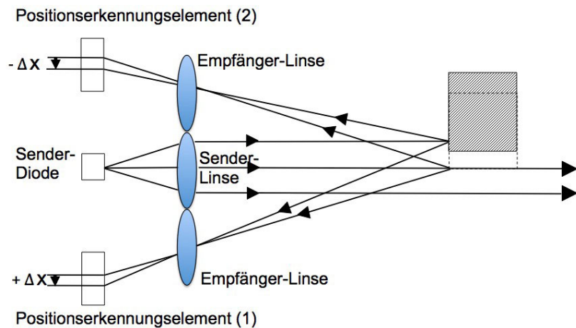
Funktionsweise der Hintergrundausblendung nach dem Dreistrahlprinzip.
