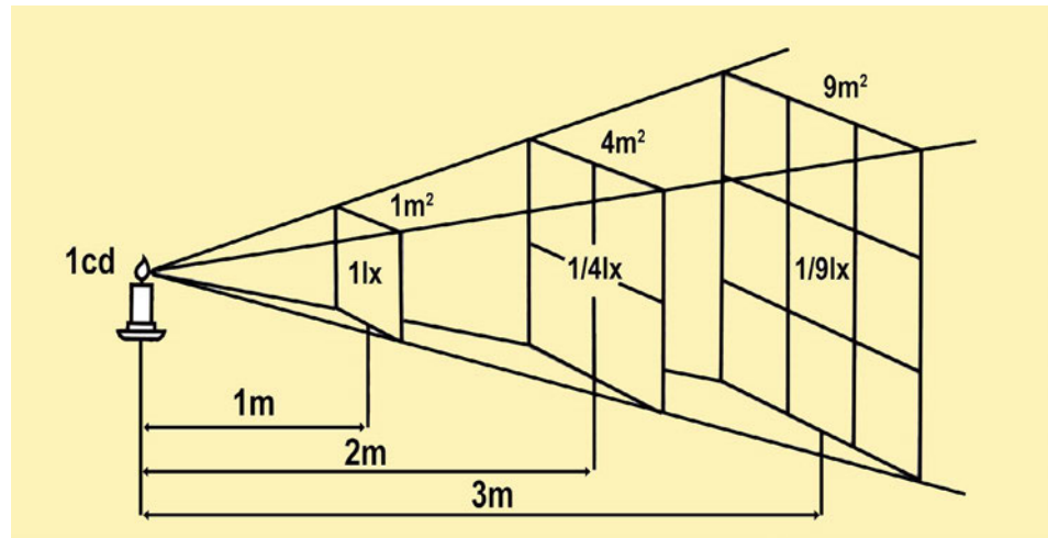
Das fotometrische Entfernungsgesetz besagt, dass die Beleuchtungsstärke mit dem Quadrat zur Lichtquelle abnimmt.
