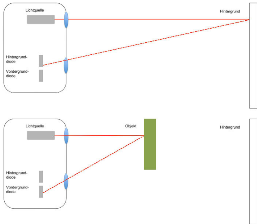
Funktionsweise der mechanischen Hintergrundaussblendung.
