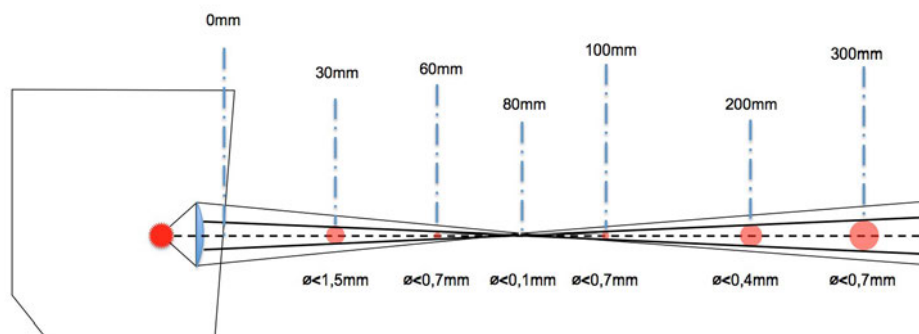
Die kleinsten Objekte können im Bereich des Laserstrahlfokus erfasst werden. An dieser Stelle ist auch die Positionier- und Wiederholgenauigkeit am größten.
