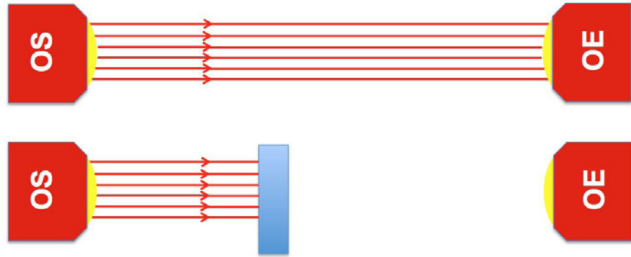
Die Einweg-Systeme werten die Lichtstrahlunterbrechung aus.
