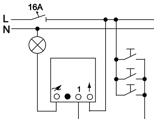
Afb. 2: Schakelschema
