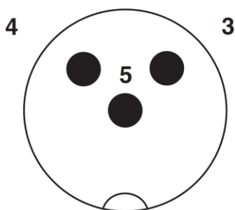
Polbild M12-Stecker, 3-polig, Ventilstecker
