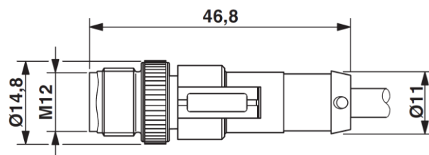
Stecker M12x1, gerade, geschirmt
