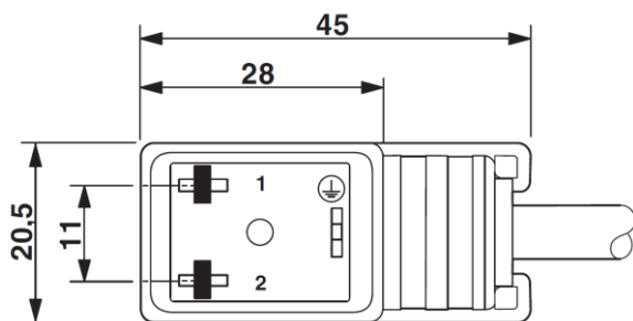
Ventilstecker Bauform BI
