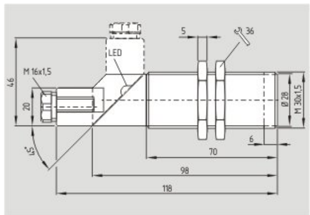
Maßzeichnung (Grundgerät)
