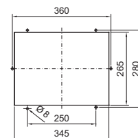
Montageausschnitt
