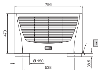
1 Kondensatablauf 1/2", flexibel
