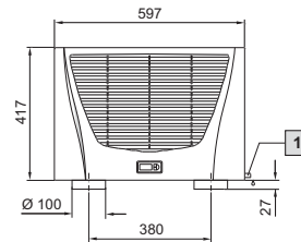
1 Kondensatablauf 1/2", flexibel
