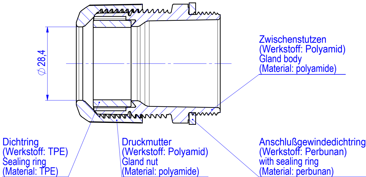
SCHNITT A-A
