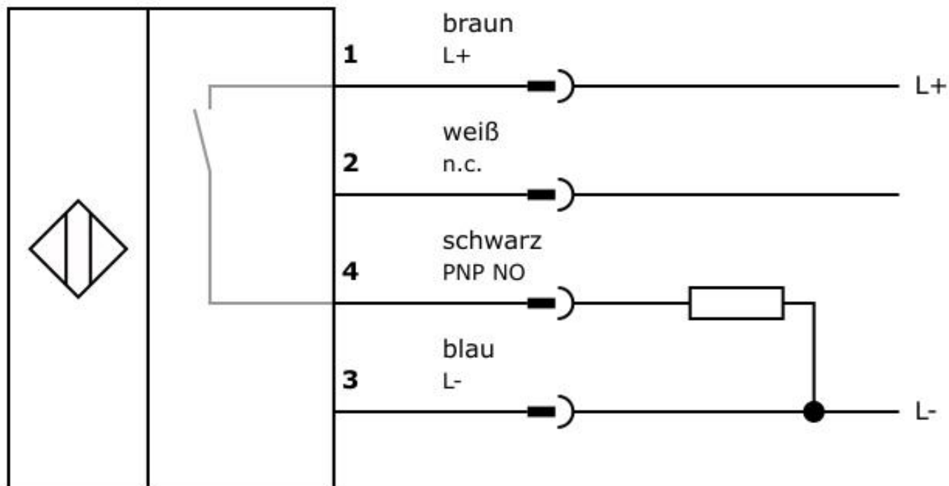
Anschlussbild
