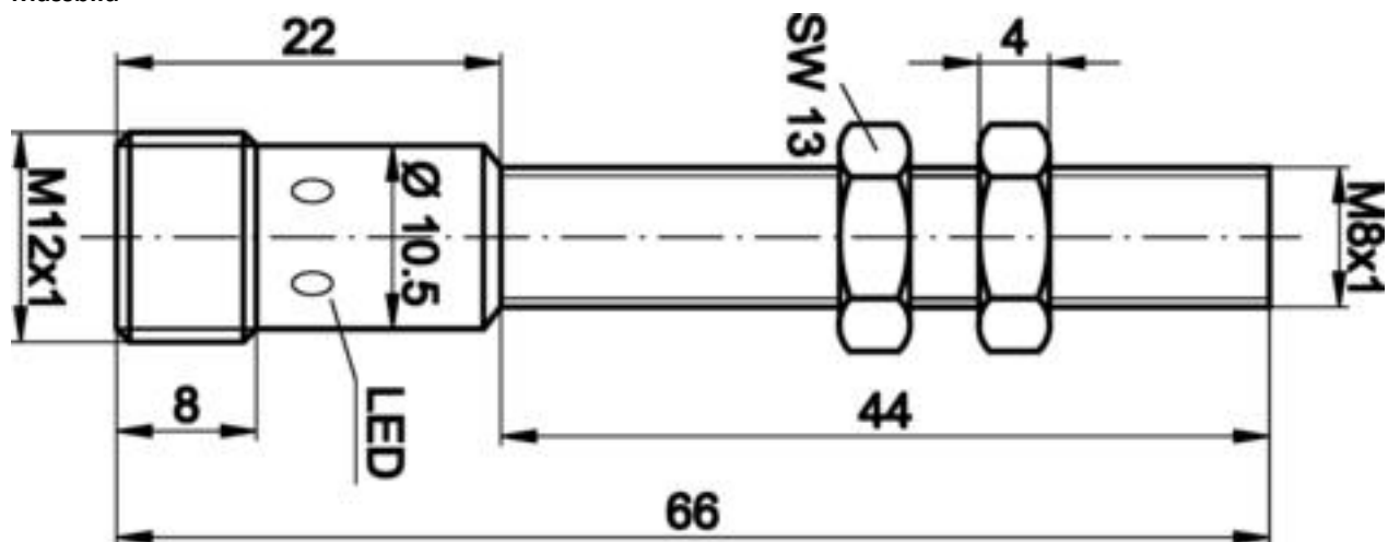
Massbild
