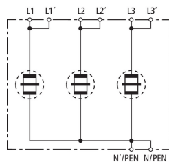
Prinzipschaltbild DB 3 255 H
