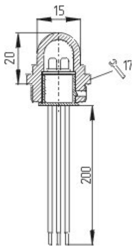
Maßzeichnung (Grundgerät)
