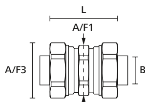
HeloGuard Kompressionsverbinder
